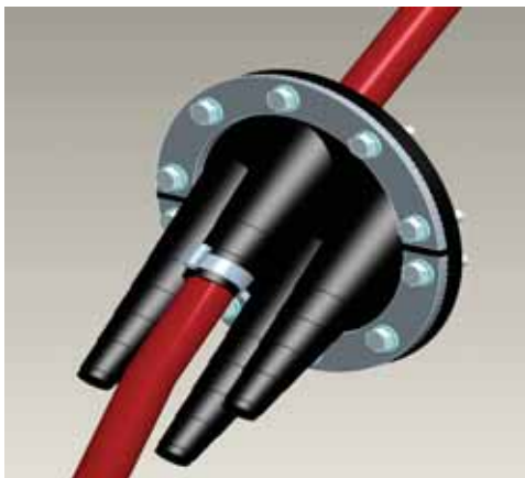
Plugs de acometida de cables en neopreno con reducción progresiva del diámetro que facilita el ruteo de cables MT y BT (vista interior dentro del centro).
